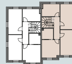
1. OBERGESCHOß
