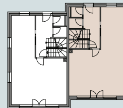
ERDGESCHOß
