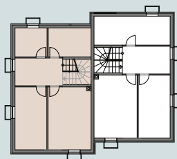
UNTERGESCHOß
