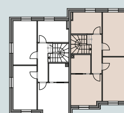
1. OBERGESCHOSS
