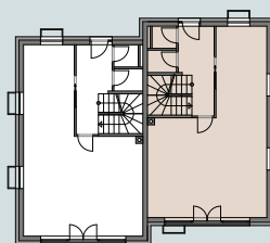
ERDGESCHOSS
