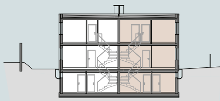
SCHNITT
