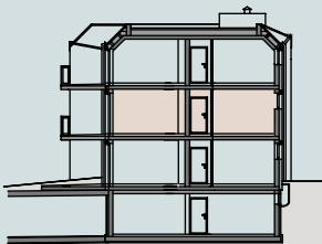
SCHNITT
