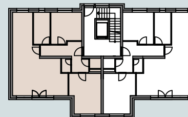
ERDGESCHOSS
