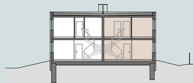
SCHNITT
