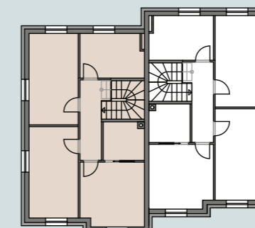
1. OBERGESCHOSS
