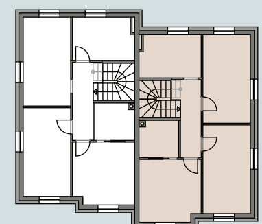
1. OBERGESCHOSS
