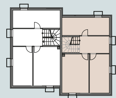
UNTERGESCHOß
