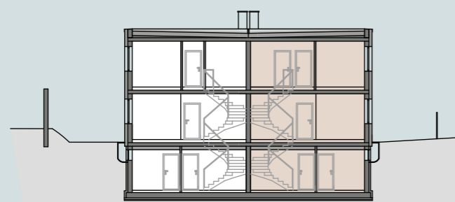
SCHNITT
