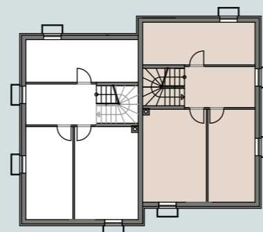
UNTERGESCHOß
