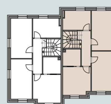
1. OBERGESCHOSS
