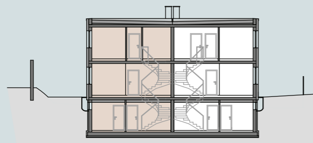
SCHNITT
