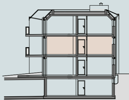
SCHNITT
